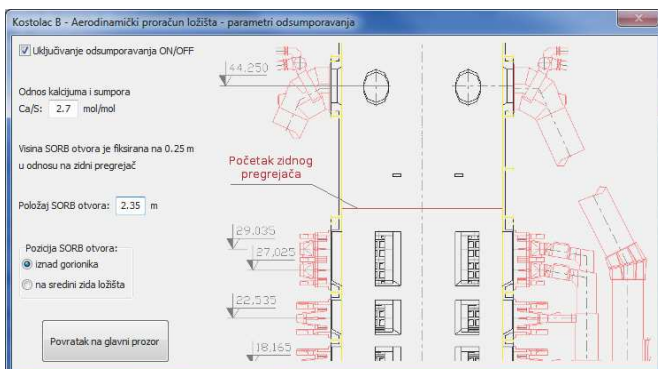
Екран за одабир параметара одсумпоравања додавањем спрашеног сорбента у ложиште
